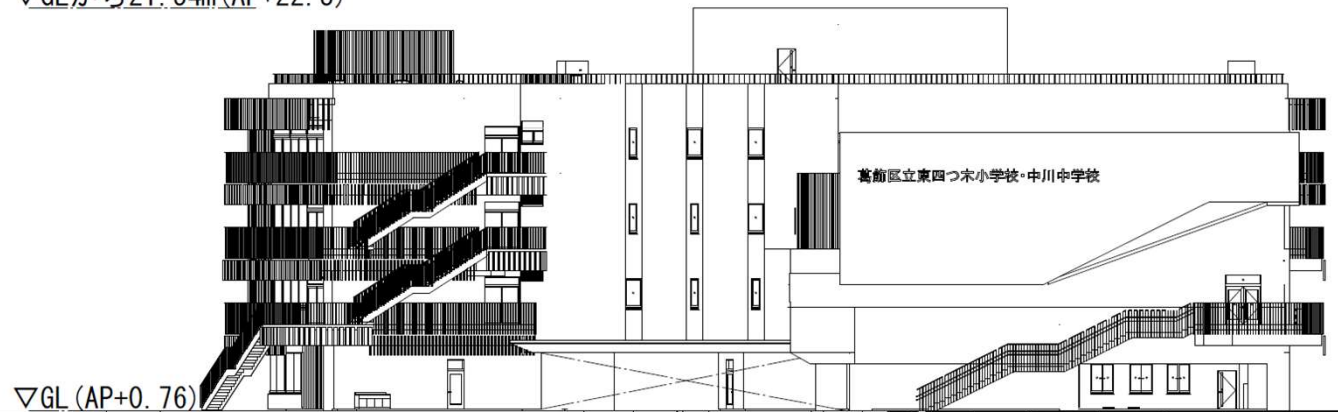
北立面図
