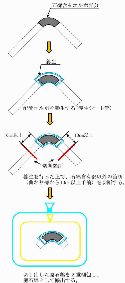
《配管エルボ部保温材(一例)》
