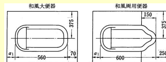
α 1 の 寸 法
