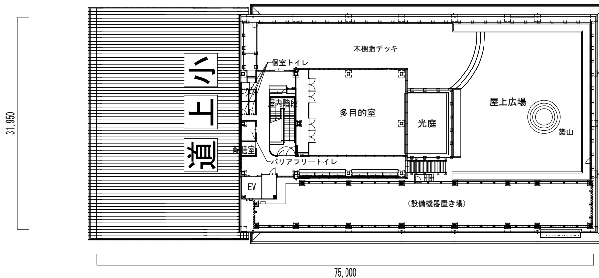
5階平面図
