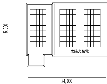
屋上平面図
