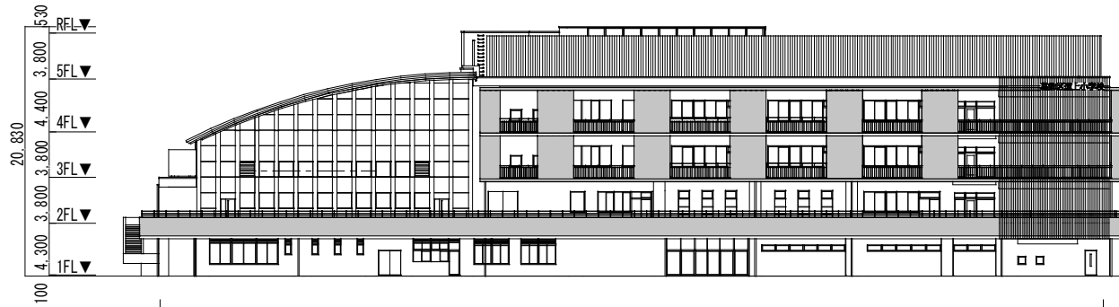
西側立面图
