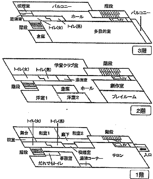
西尾久ふれあい館のレイアウト図
